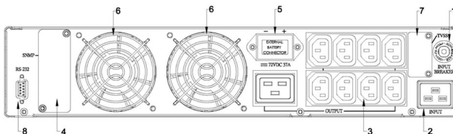
Рис. 2-6.2. Задняя панель ИБП на 2 и 3 кВА
