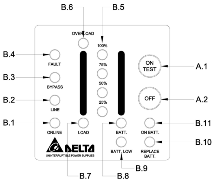
Рис. 2-5. Панель управления
