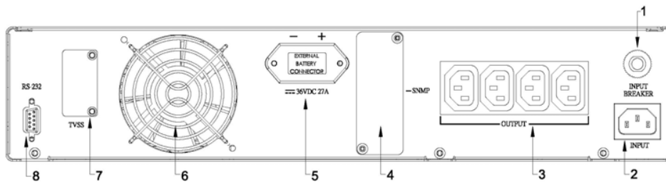
Рис. 2-6.1. Задняя панель ИБП на 1 кВА
