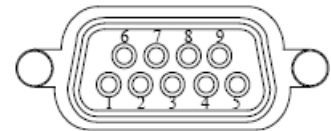
Рис. 8-1 Назначение контактов
