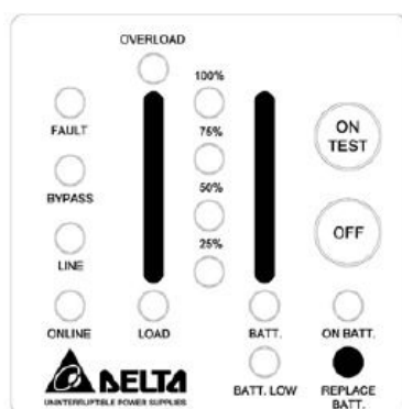
Рис. 4-6. Индикация необходимости замены батареи
