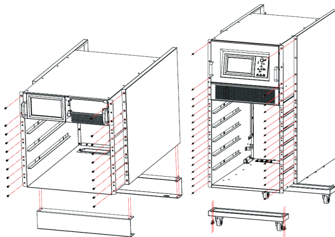
(а) Снимите боковые панели и держатели
