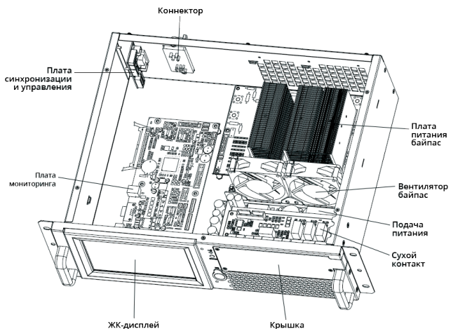
(a) Модуль статического байпаса 20/40 кВА
